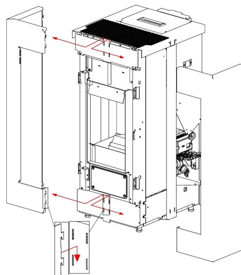
Fig. 30 - De zijpanelen losmaken
