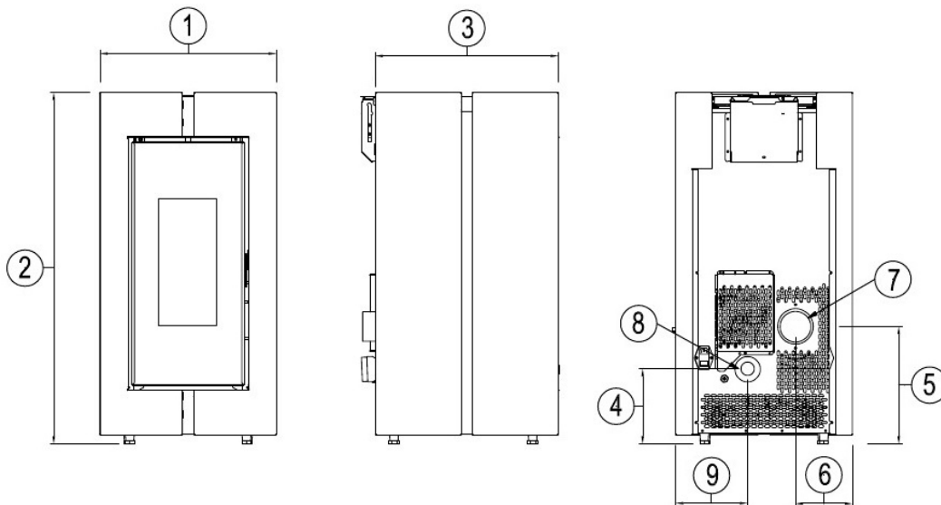
Fig. 15 - Algemene afmetingen: Tecna 3
