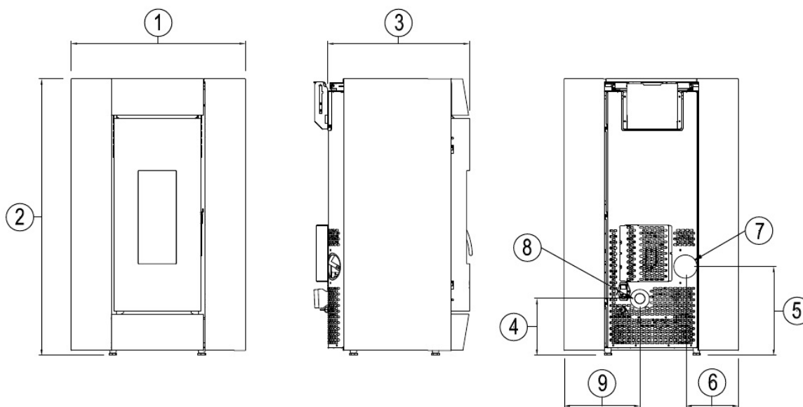
Fig. 18 - Algemene afmetingen: Elise 3
