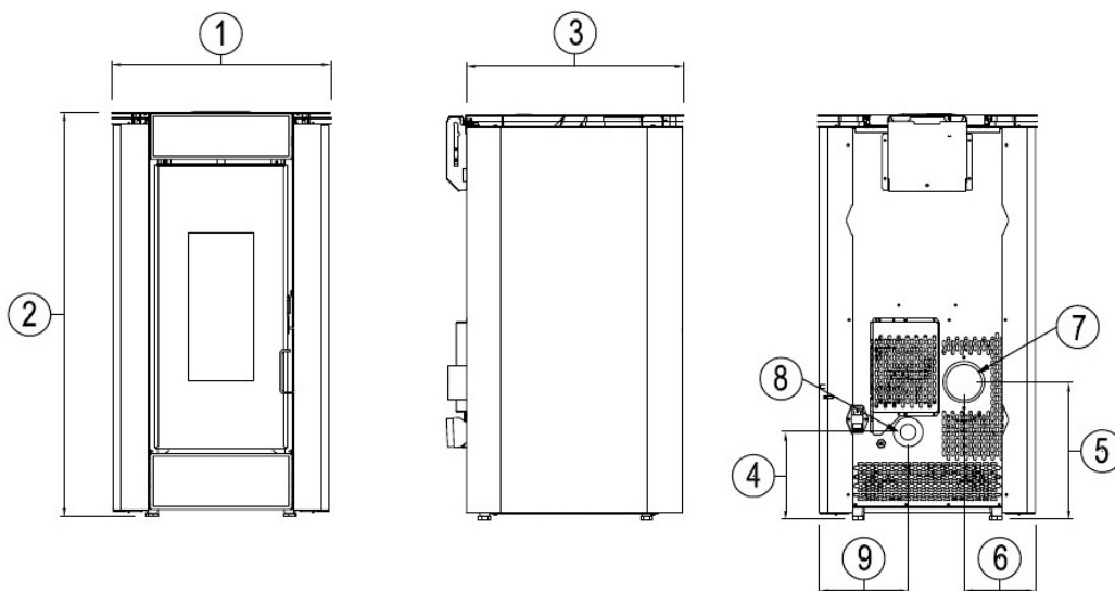
Fig. 16 - Algemene afmetingen: Evo 3
